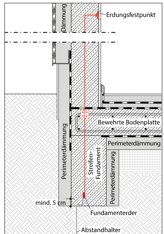
Bild 26: Ausführung des Fundamenterders bei beidseitiger Anordnung der Perimeterdämmung an einem Streifenfundament
