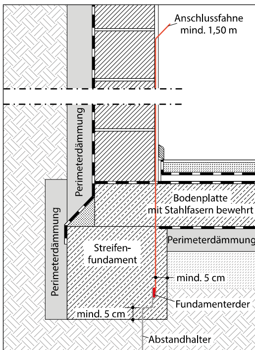
Bild 24: Ausführung des Fundamenterder bei einseitiger Anordnung der Perimeterdämmung an einem Streifenfundament
