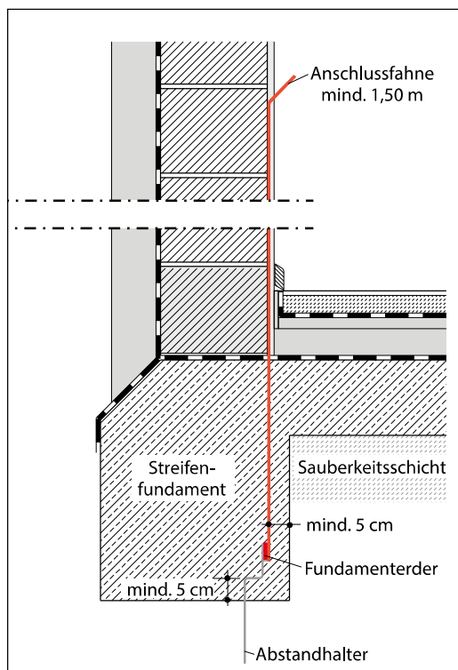
Bild 14: Ausführung eines Fundamenterders im unbewehrten Fundament
